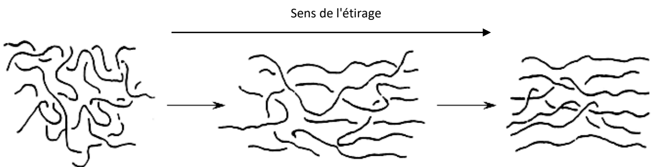
Étirage uni-axial d'un polymère amorphe
