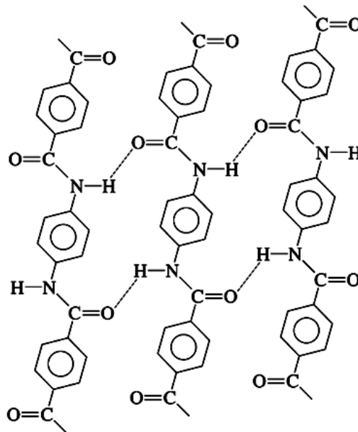
Liaisons hydrogène entre les chaînes du polyamide (le Kevlar®)
